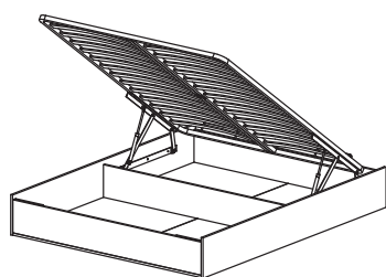
Бельевой ящик для кровати 160x200 с подъёмным механизмом Размеры (ШхВхГ): 1610x280x2005
