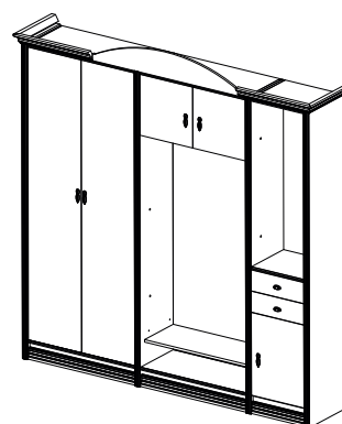
Прихожая №3 Размеры (ШхВхГ): 2175x2240x415
