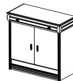
Тумба №10 Размеры (ШхВхГ): 865x815x400
